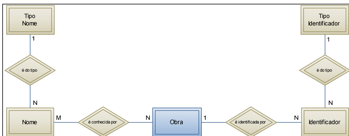
Figura 56 – Estendendo o modelo com entidades FRAD
