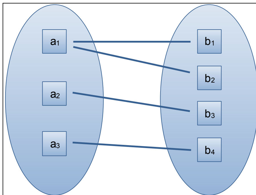
Figura 16 – Relacionamento um-para-muitos
