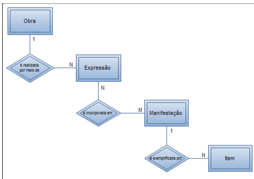
Figura 51 – Modelo Conceitual com as Entidades do Grupo 1
