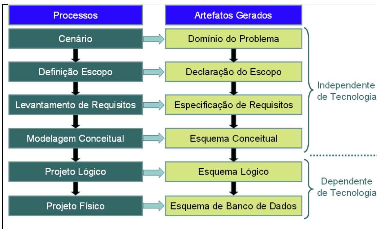
Figura 11 – O processo de modelagem de dados
