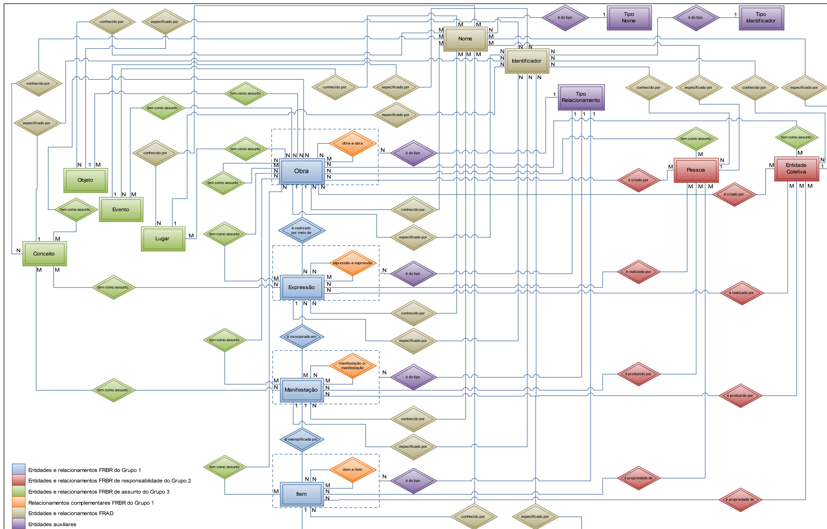
Figura 57 – Modelo conceitual baseado nas entidades e relacionamentos dos FRBR e FRAD
