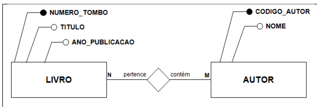
Figura 13 – Diagrama Entidade-Relacionamento
