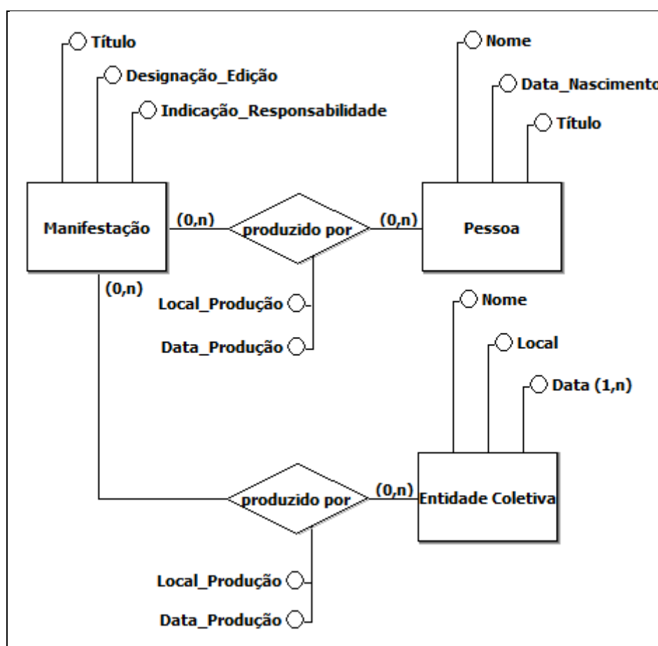
Figura 27 - Diagrama Entidade-Relacionamento
