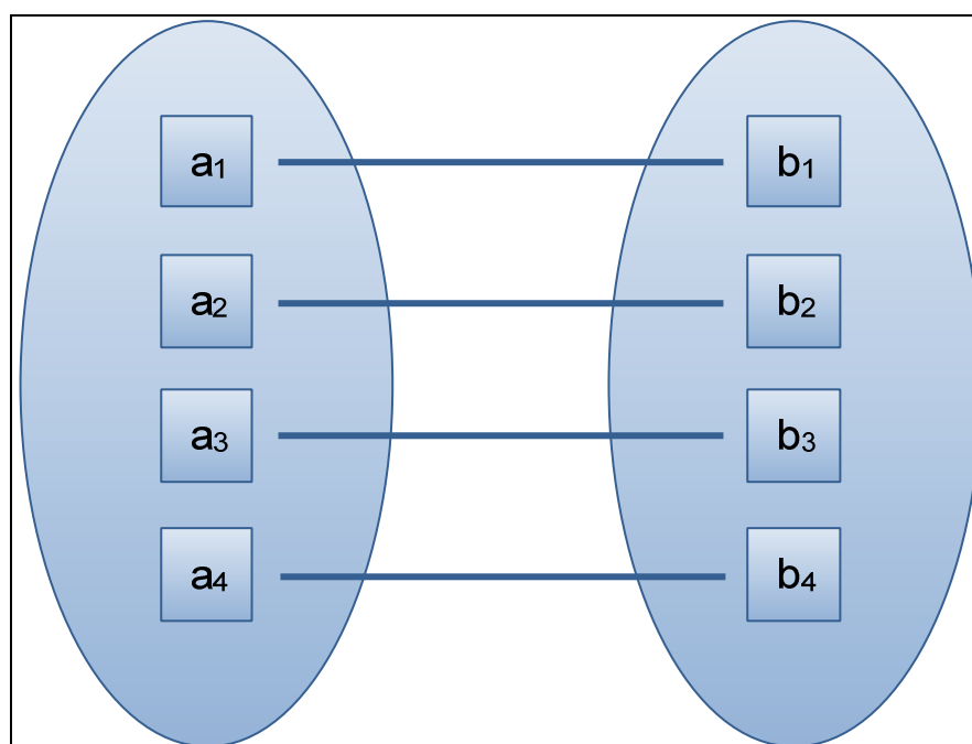
Figura 14 – Relacionamento um-para-um
